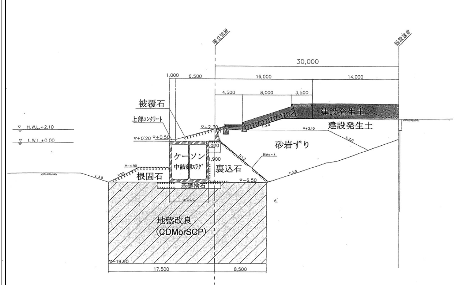
ケーソン式護岸 (標準断面図)
