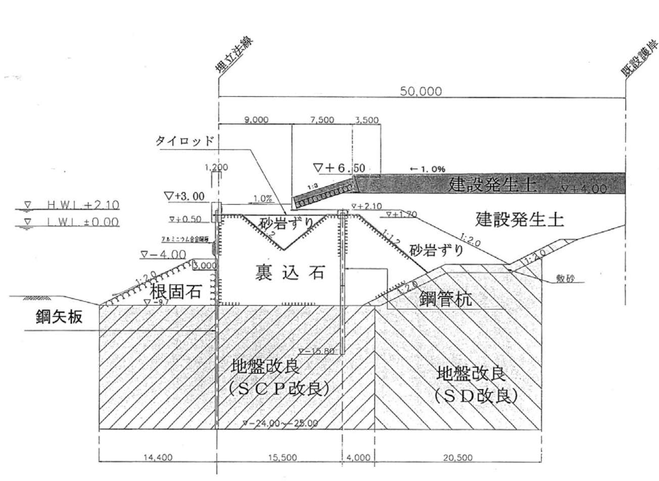
鋼矢板控え式護岸 (標準断面図)
